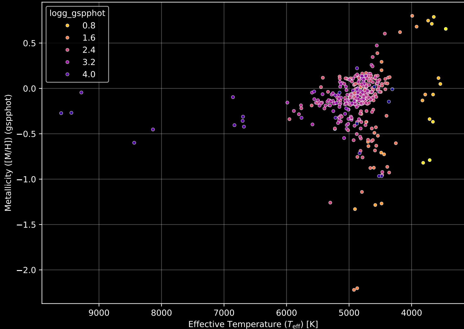
APOGEE DR17 Field: [010-12] Stellar Population Parameters (n= 379)
